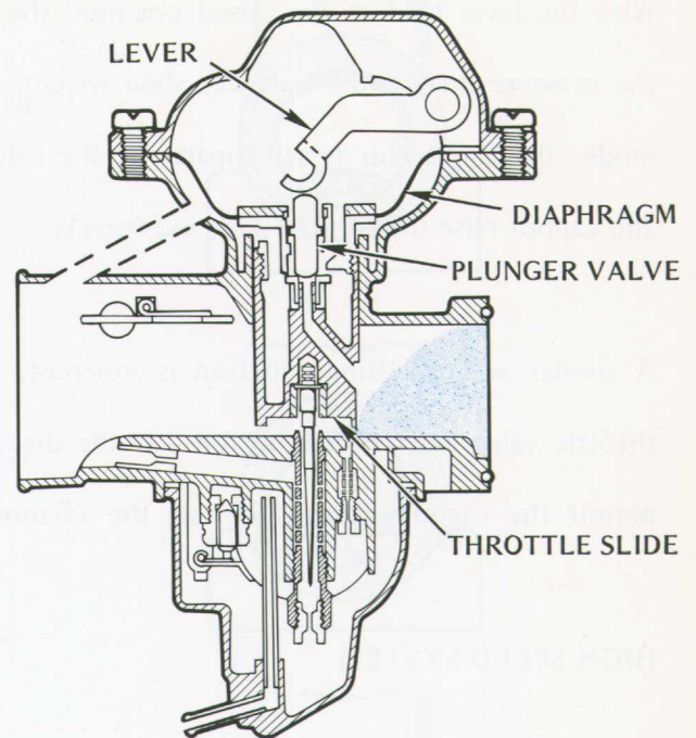
FIG. 37 Idle Position
